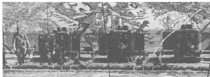
So sieht eine Feldpipeline-Hochdruckstation im Betrieb aus: Die Leistung liegt bei 300 000 Litern Kraftstoff pro Stunde.
